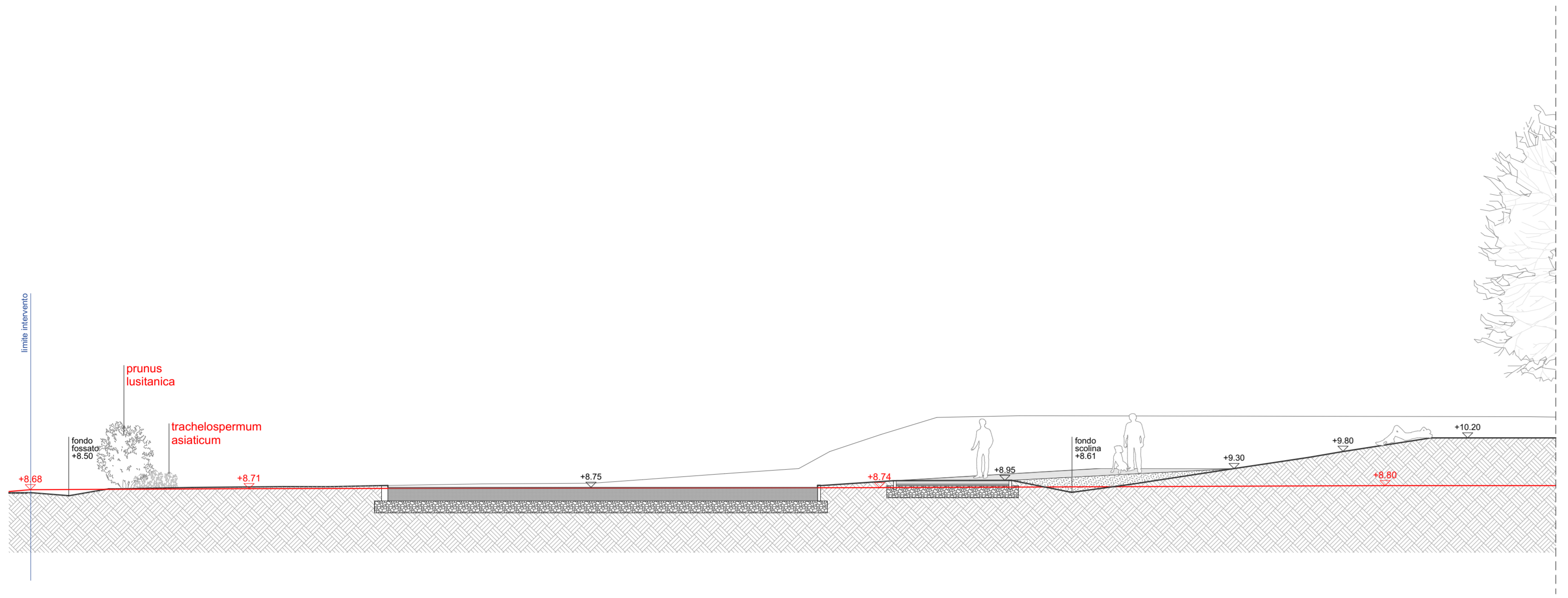
SEZIONE A-A' - scala 1:100
